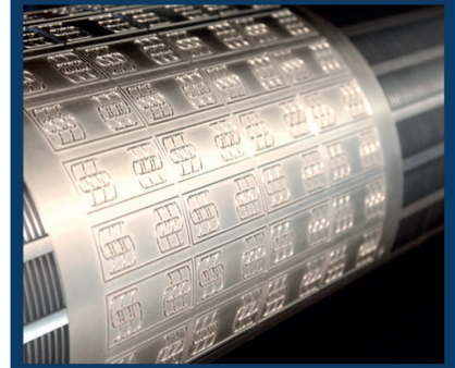
Etikettenstanzblech
